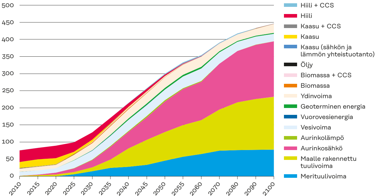
Kuva 3: Sähköntuotanto (pääskenaario)
