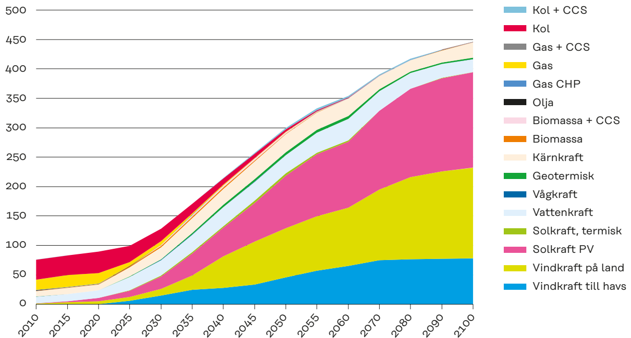
Figur 3: Elproduktion (centralt scenario)
