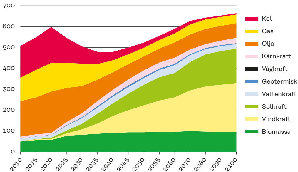
Figur 3: Elproduktion (centralt scenario)
